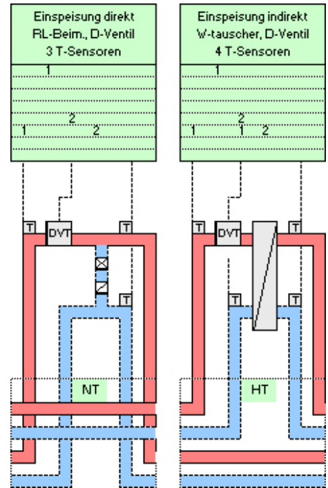
Bild 39 Einspeisung direkt
