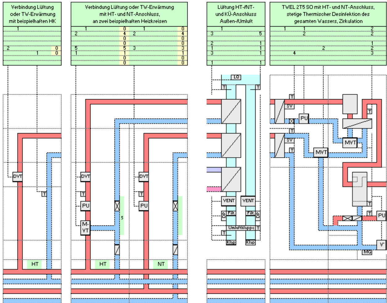
Bild 36.2 HK T-Regelung
