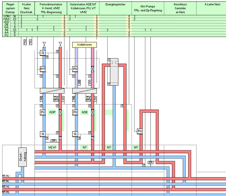
Muster Bild 1 HA-System Wärmeerzeugung mit FW- Station mit NW-Pumpe, Solarstation mit E-Speicher und NW-Pumpe, Netz DP positiv
